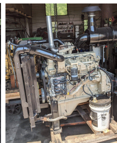
Cummins QSB 6.7
